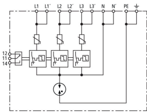
Schema di principio DCU EMOB 2 25
