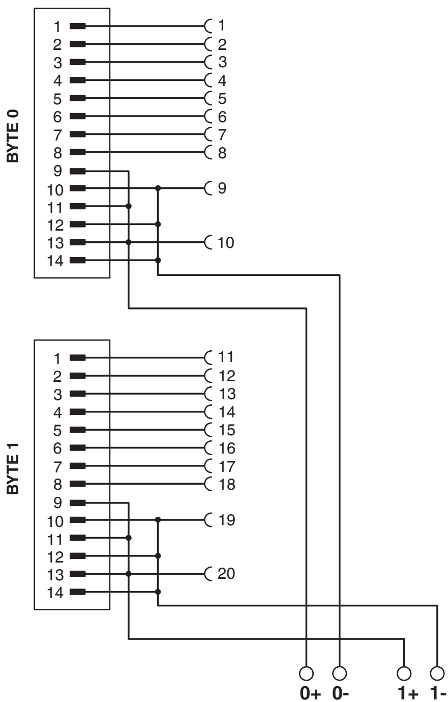
Diagrama eléctrico
