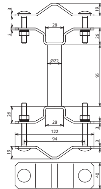
Maßbild BSC D40 DS95 D45.65 V2A
