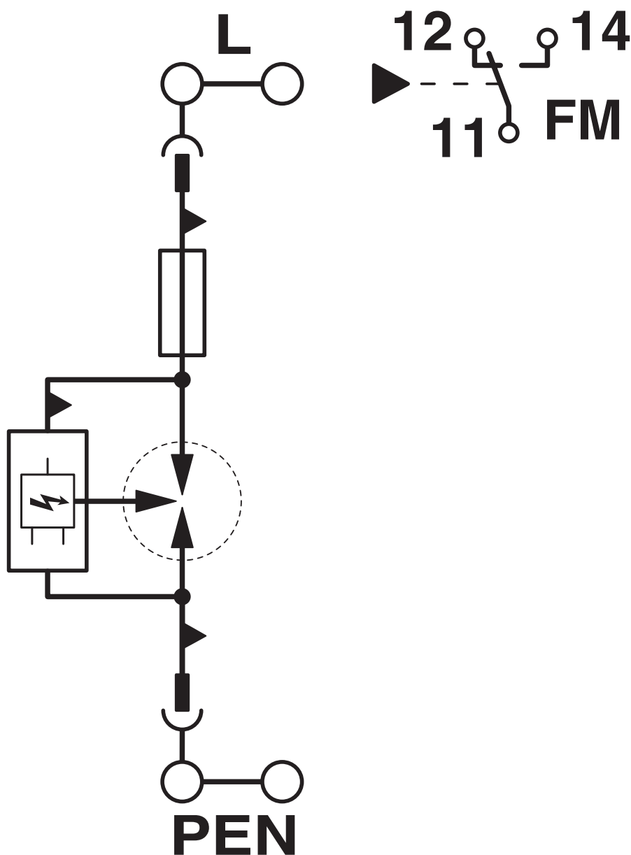
Diagrama eléctrico
