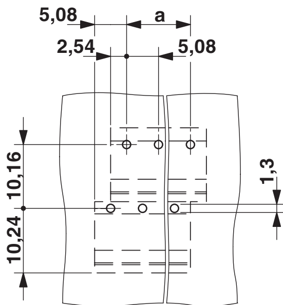
Bohrplan/Lötpadgeometrie
