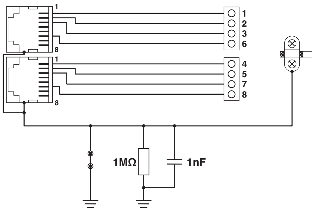
Diagrama eléctrico
