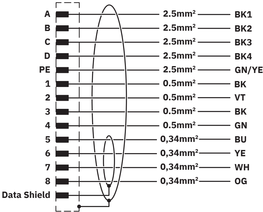
Diagrama eléctrico
