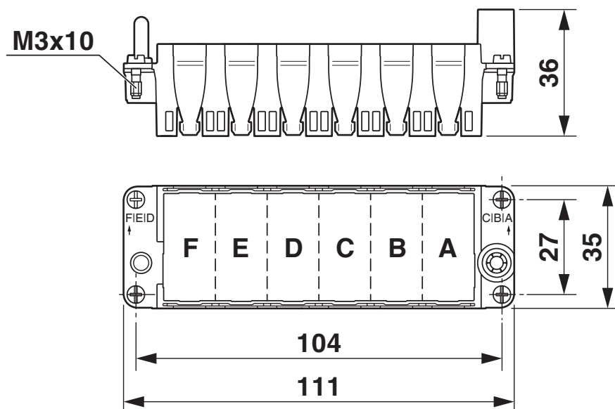
Dessin coté
