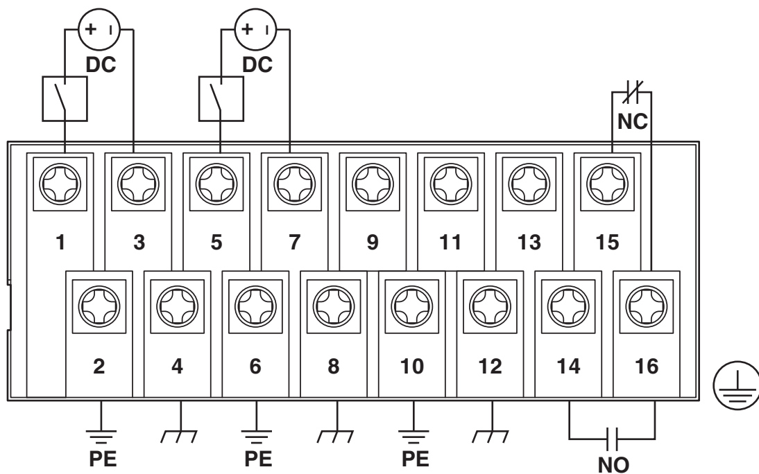
Anschlusszeichnung
