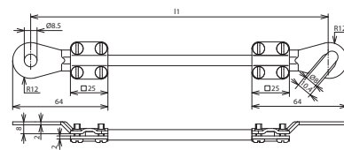
Maßbild EL10 L1.05M 1KSO 8.10 1KSG 8
