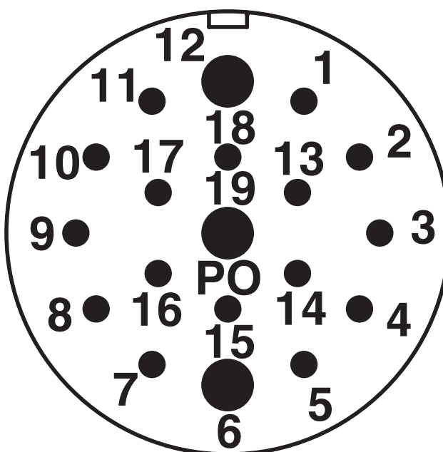
Plano esquemático
