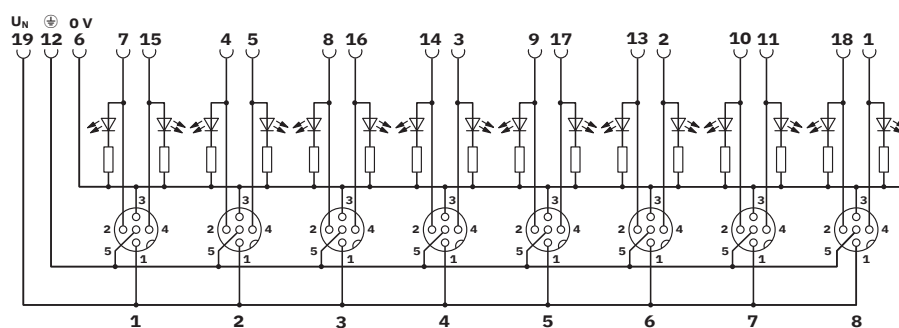
Diagrama eléctrico
