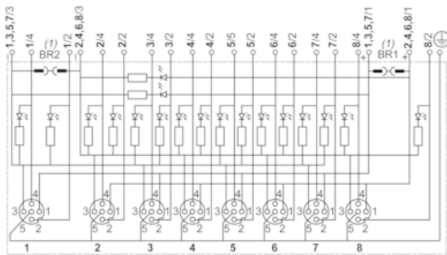
(1) BR1 y BR2: conexión extraíble
