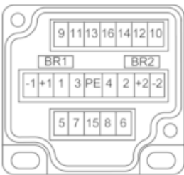
Terminales de conexión
