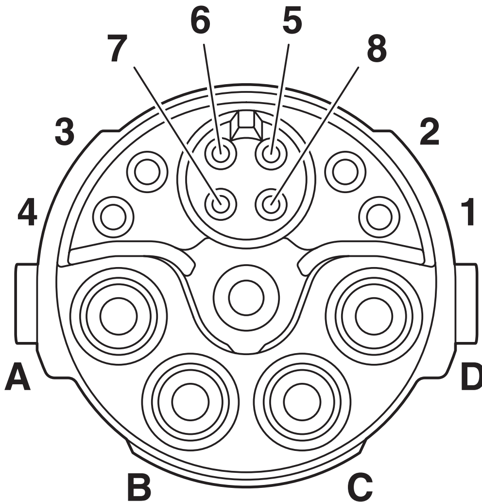
Schemazeichnung
