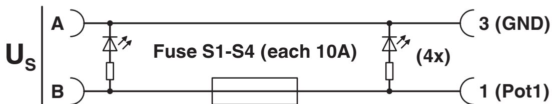
Diagrama eléctrico
