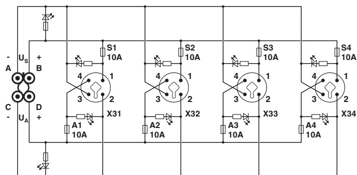
Diagrama eléctrico
