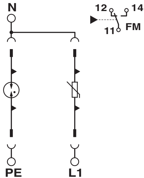
Diagrama eléctrico
