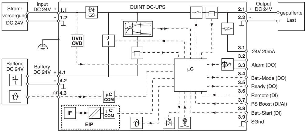
Blockschaltbild
