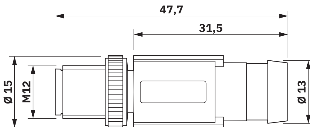
Dessin coté
