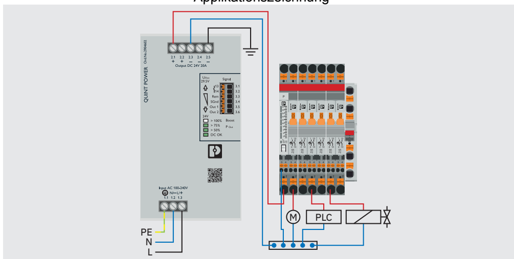
Applikationszeichnung
