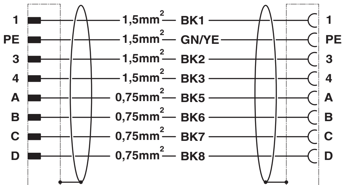
Diagrama eléctrico
