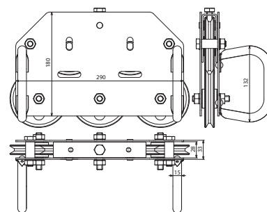
Maßbild DRG 5RO 7.10 HG STGALZN
