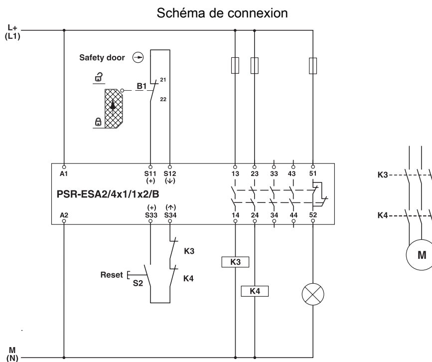
Surveillance de porte de protection monocanal
