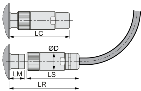
Gerade Stecker
