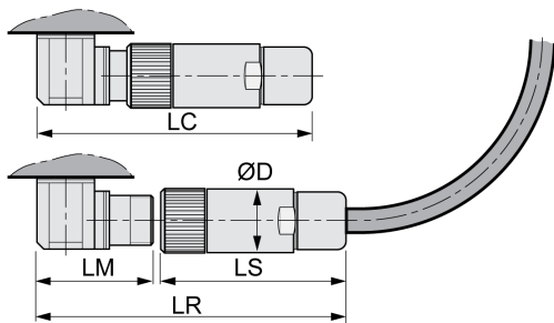
Winkelstecker
