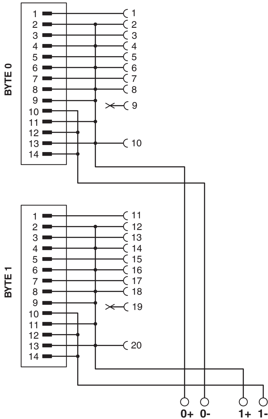
Diagrama eléctrico
