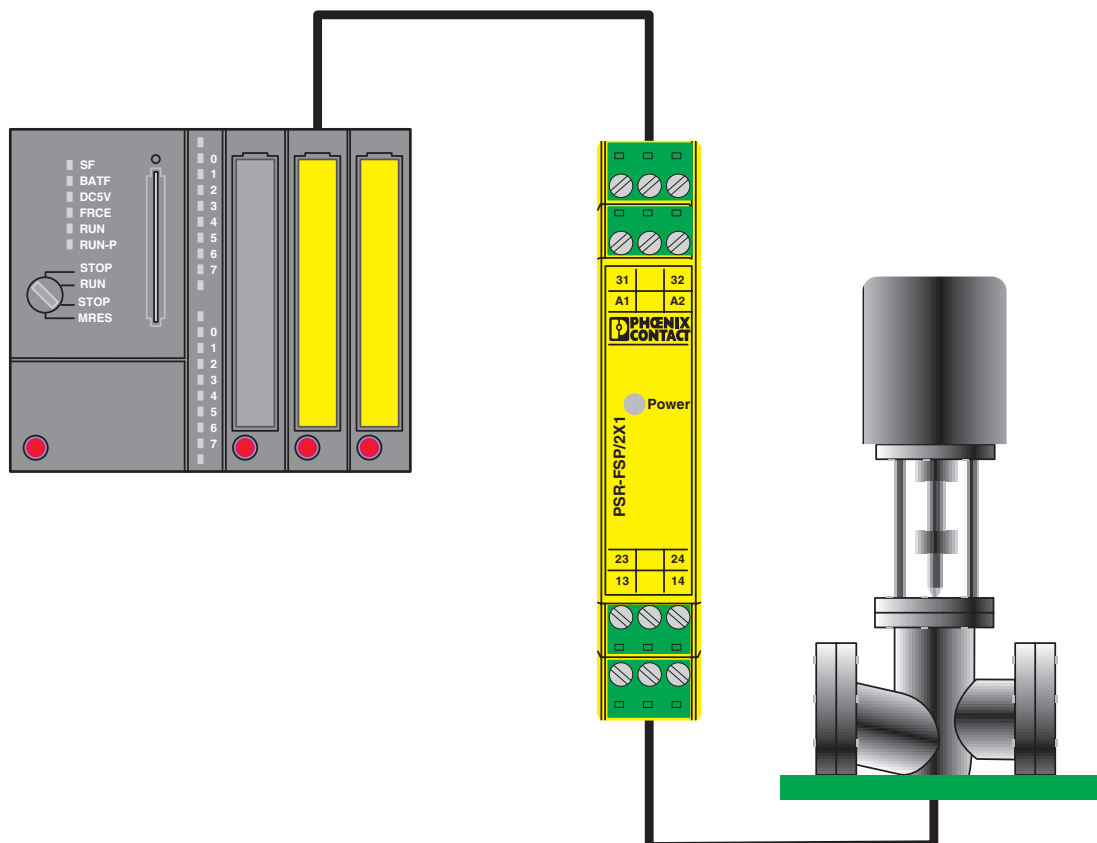
Applikationszeichnung
