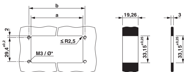
Esquema de dimensiones
