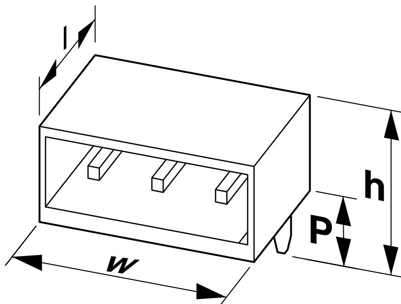
Dessin coté
