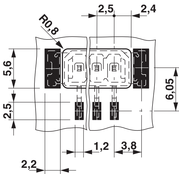
Bohrplan/Lötpadgeometrie
