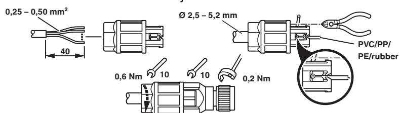
Dibujo funcional
