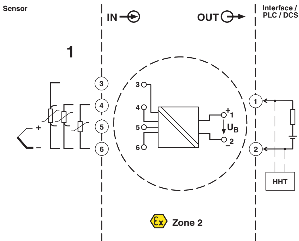
Blockschaltbild
