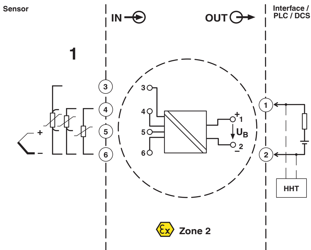
Schéma fonctionnel
