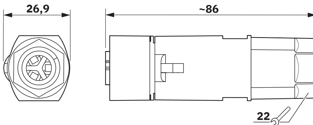
Dessin coté
