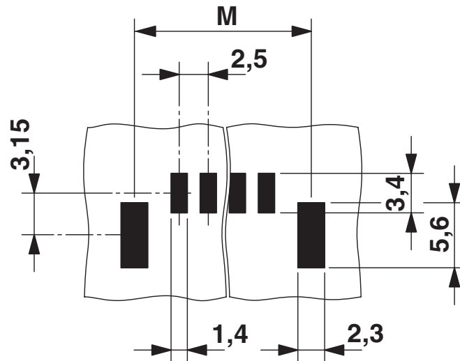
Bohrplan/Lötpadgeometrie
