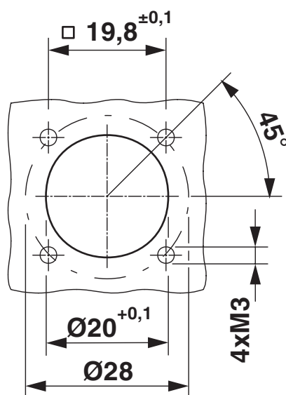
Plano esquemático
