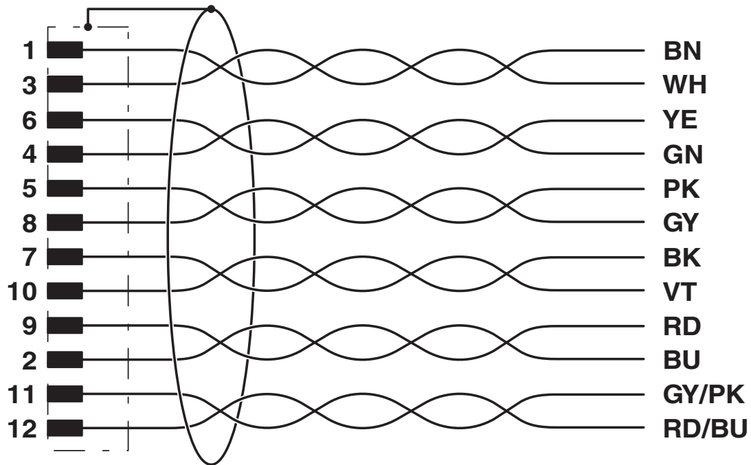
Diagrama eléctrico
