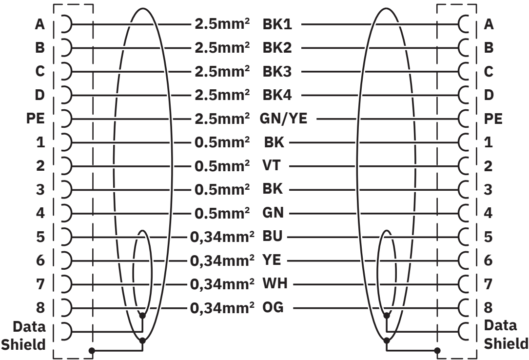
Diagrama eléctrico
