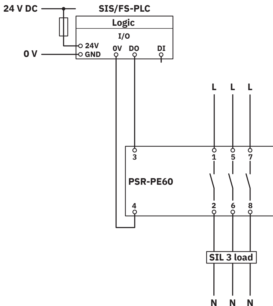
Diagrama eléctrico
