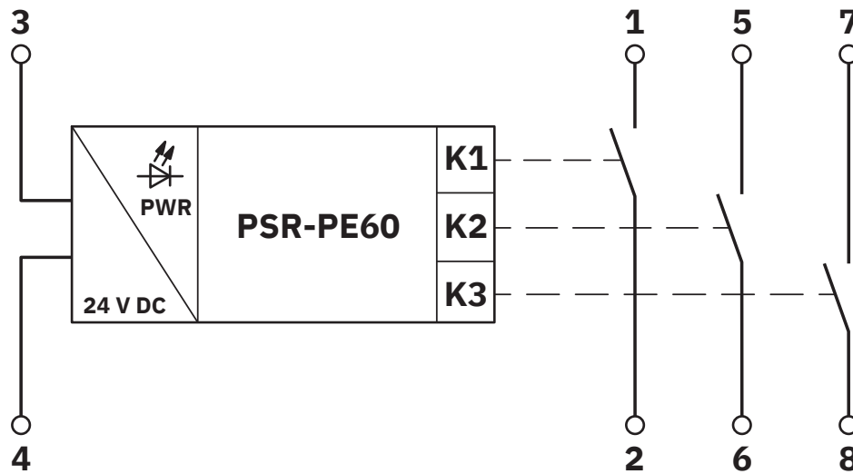
Schéma fonctionnel
