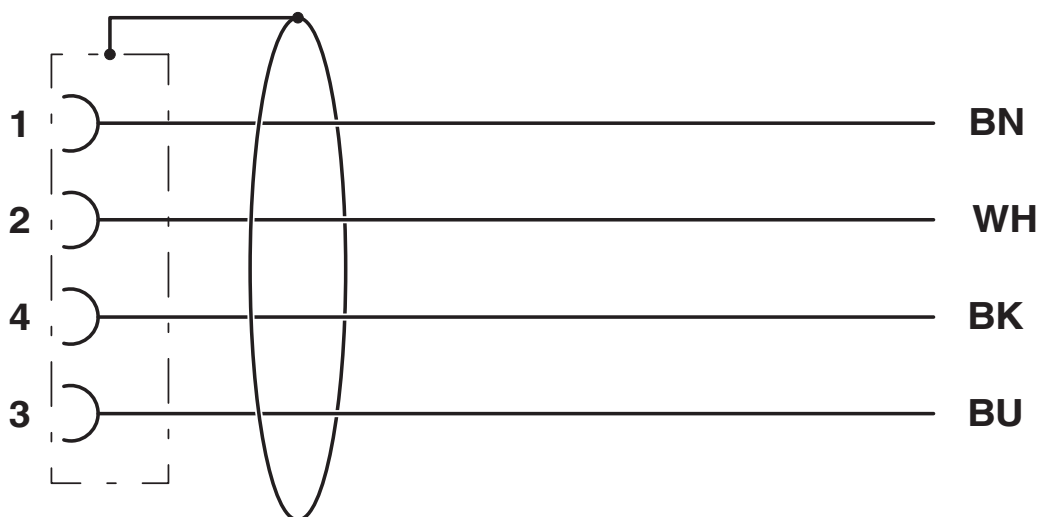
Ocupación de contactos del conector hembra M8
