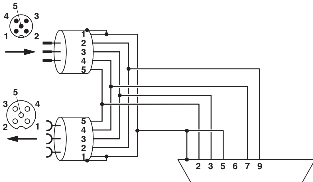
Diagrama de contactos de función SUBCON-PLUS-CAN/...M12
