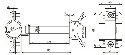
Maßbild LH ZS 27 EX P85 SBB V2A
