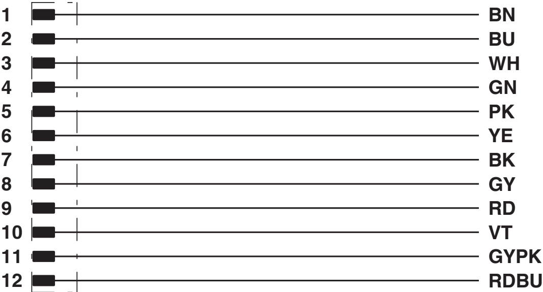
Diagrama eléctrico
