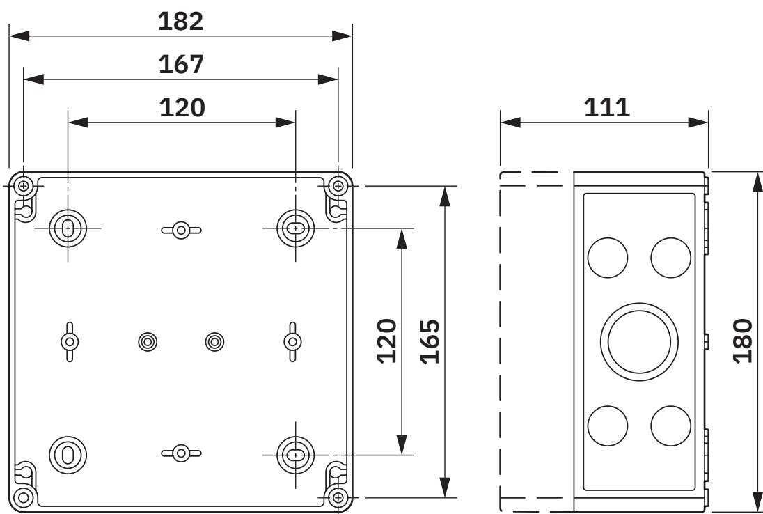
Dimensions du boîtier
