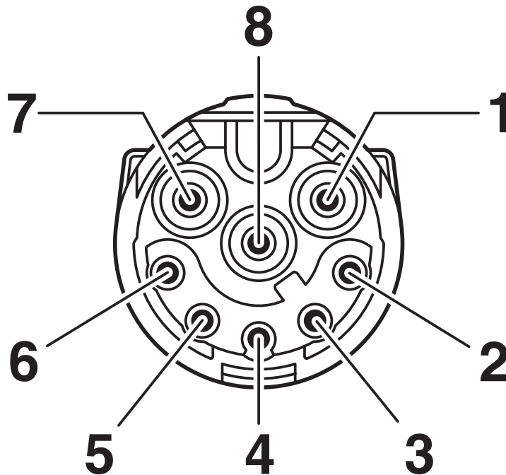
Schemazeichnung
