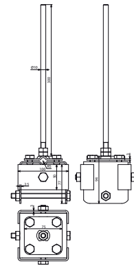
Maßbild SPK 100X100 FSP10 300 7.10 V2A
