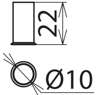
Maßbild AEH 50 L22 CUGALSN
