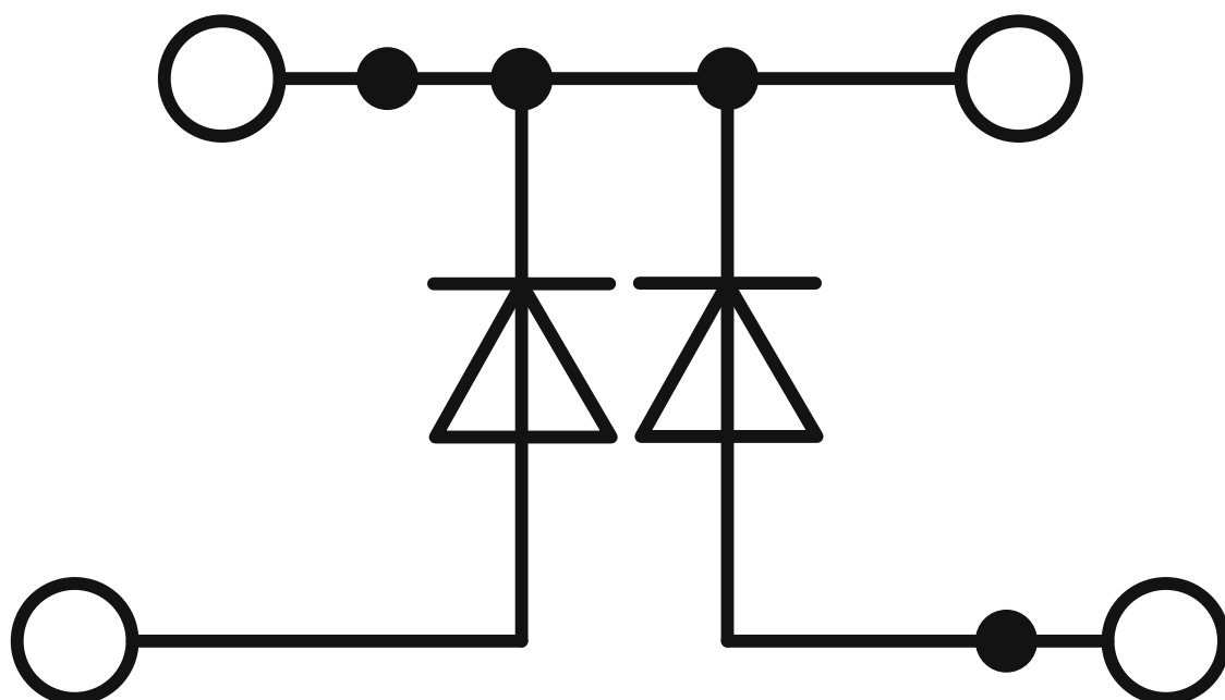
Diagrama eléctrico
