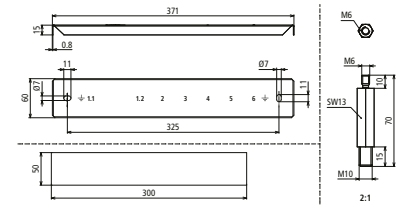
Maßbild PAS EX AD 7 AP
