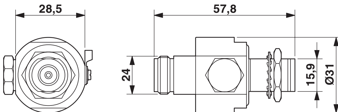
Esquema de dimensiones CN-UB-280DC-3-BB
