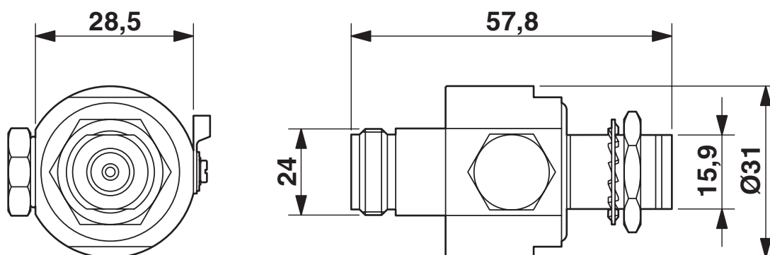
Dessin coté
