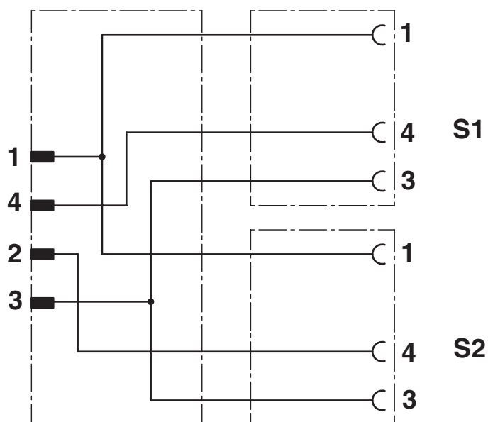
Ocupación de contactos del conector macho M8 y del conector hembra M8
